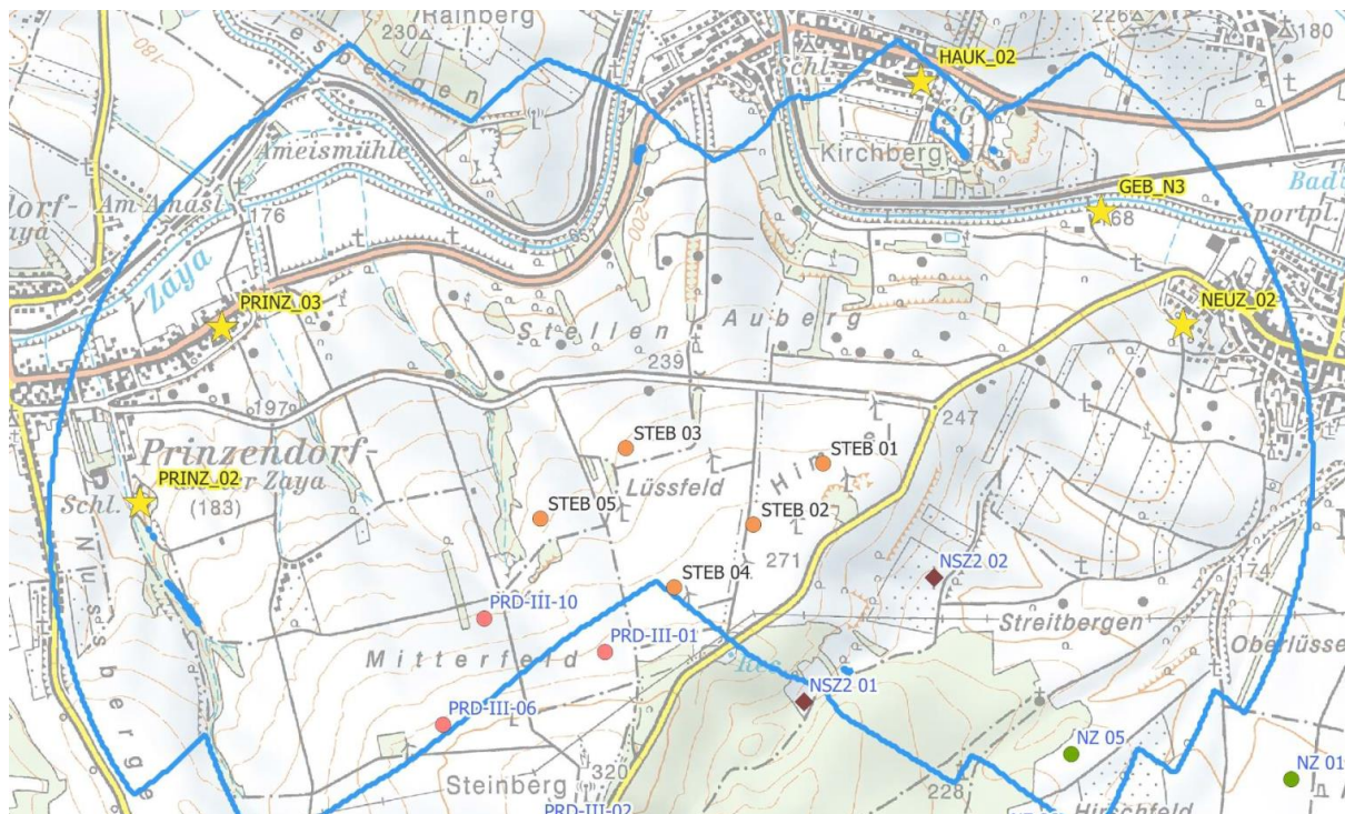
Betrachtete Immissionspunkte beim Schattenwurf
