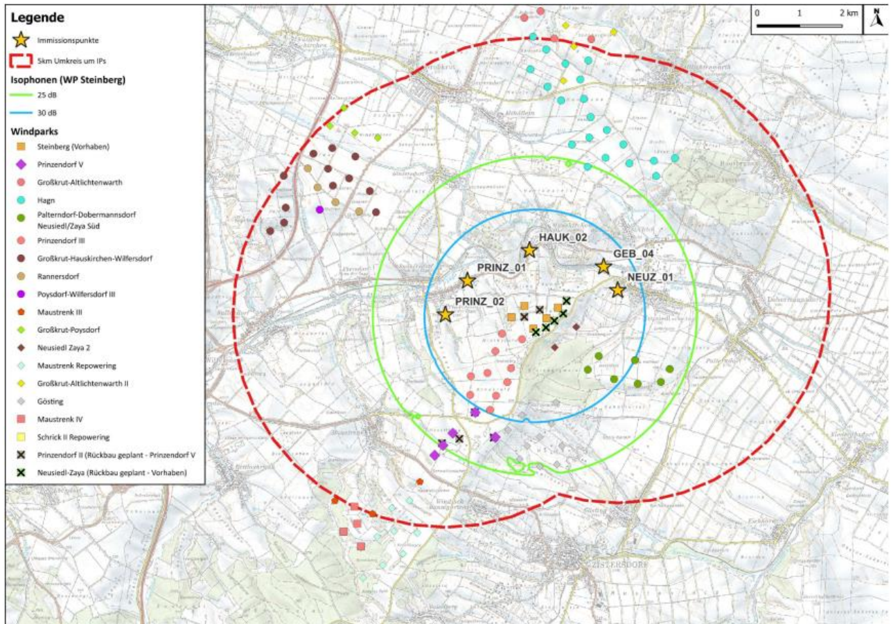
Abbildung 1: Schallimmissionen verursacht durch den geplanten Windpark Steinberg (Einlage D.03.02.00-01).
