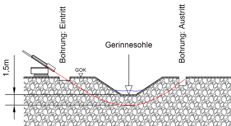
Abbildung 11: Schematische Darstellung Spülbohrung
