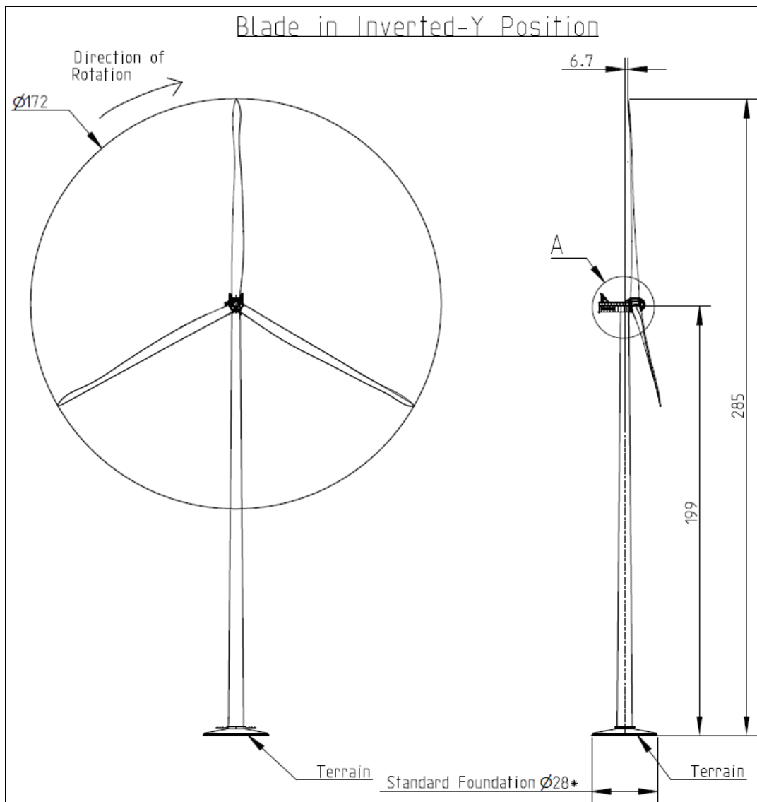
Abbildung 1: Front- und Seitenansicht der Vestas V172-7.2MW auf 199 m NH, Quelle: Fa. Vestas
