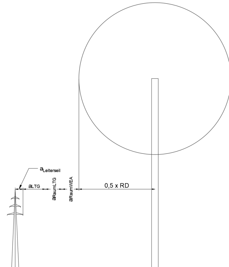
Abbildung 10: Schematische Darstellung Abstände gem. OVE EN 50341-2-1; 2023-01-01 (Eigene Darstellung)
