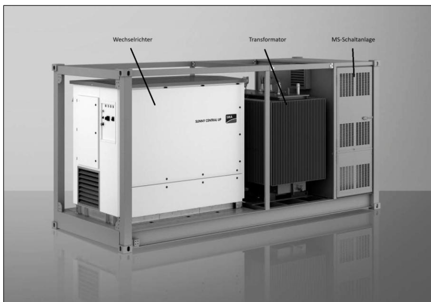
Abbildung 7: MVPS Skizze (Quelle SMA)
