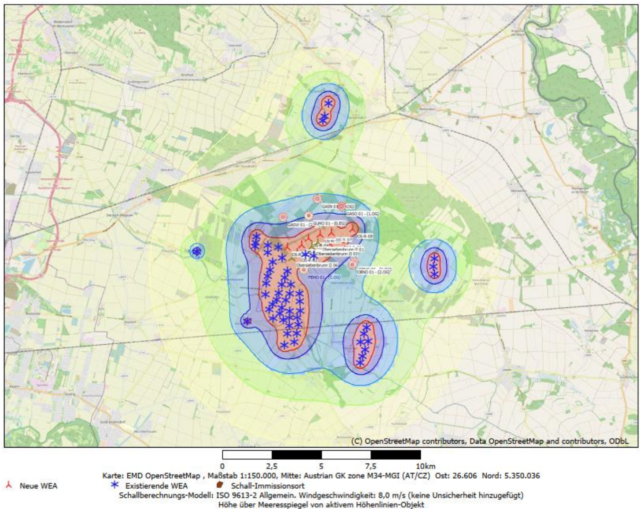
Abbildung 1: Karte der Lärmimmissionen ( v=8 m/s) inklusive benachbarte Windenergieanlagen.
